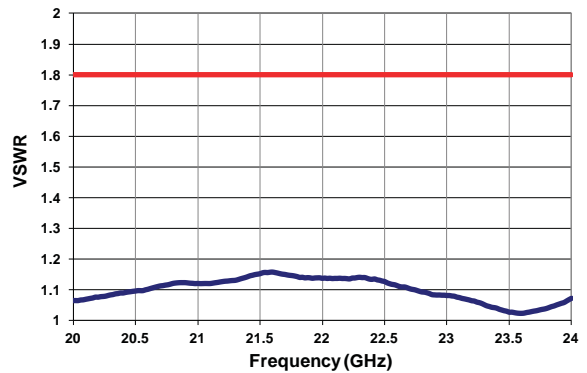
VSWR ( 20-24 GHz )
