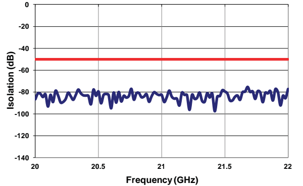
Isolation (20-22 GHz)
