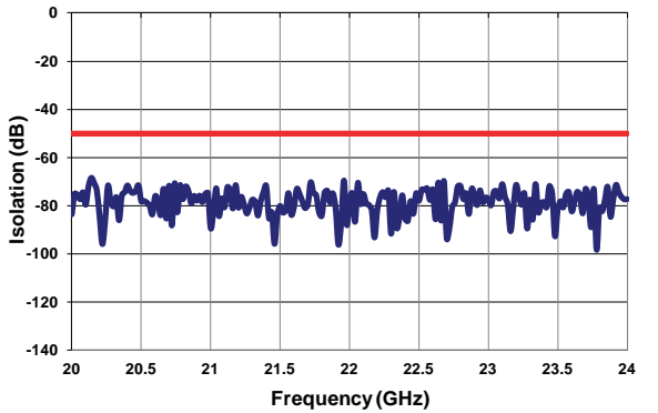
Isolation (20-24 GHz)
